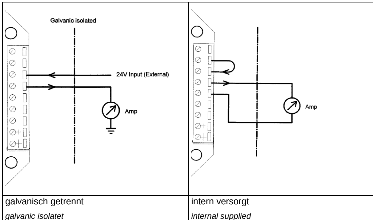
Abbildung 5: Anschluss 4-20mA Stellungsrückmeldung (optional)
