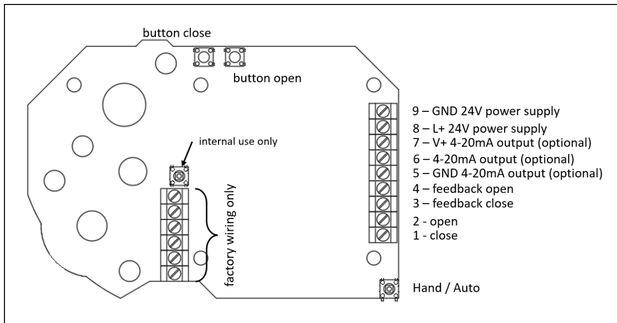
Abbildung 4: AB380 Anschlussbild
