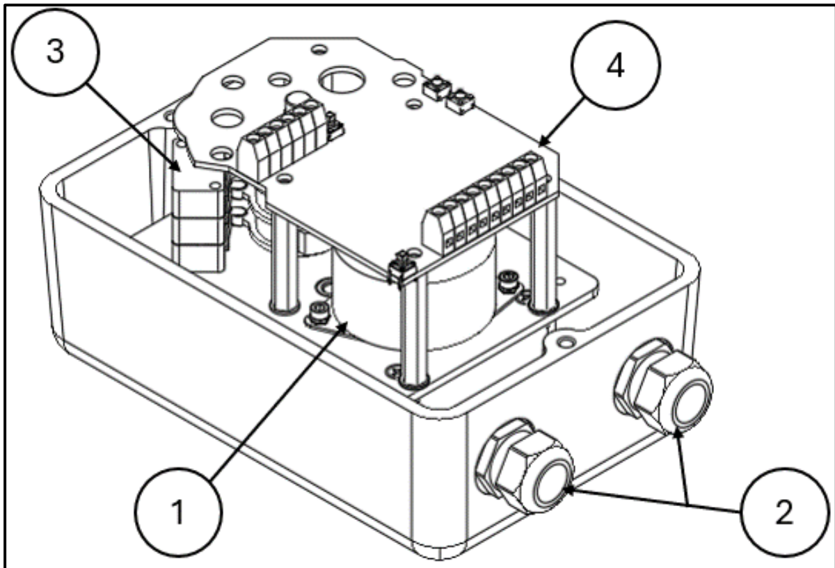
Abbildung 1: Geräteübersicht 02-25 AB380-Platine, stellvertretend für alle Antriebsserien
