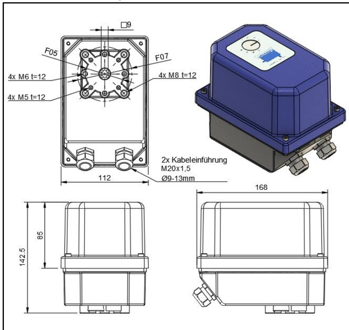
Abbildung 8: Abmessungen Antrieb Typ 01-15
