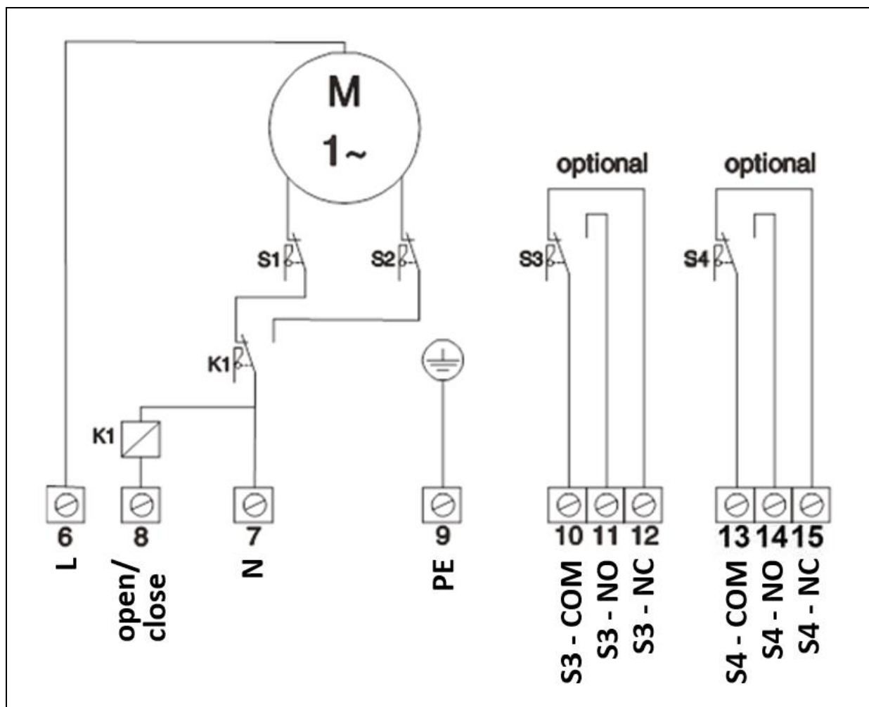
Abbildung 6: AB177 Stromlaufplan
