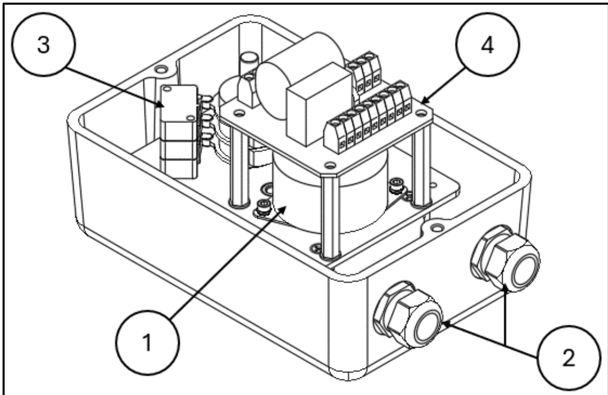
Abbildung 1: Geräteübersicht 02-25 AB177-Platine, stellvertretend für alle Antriebsserien
