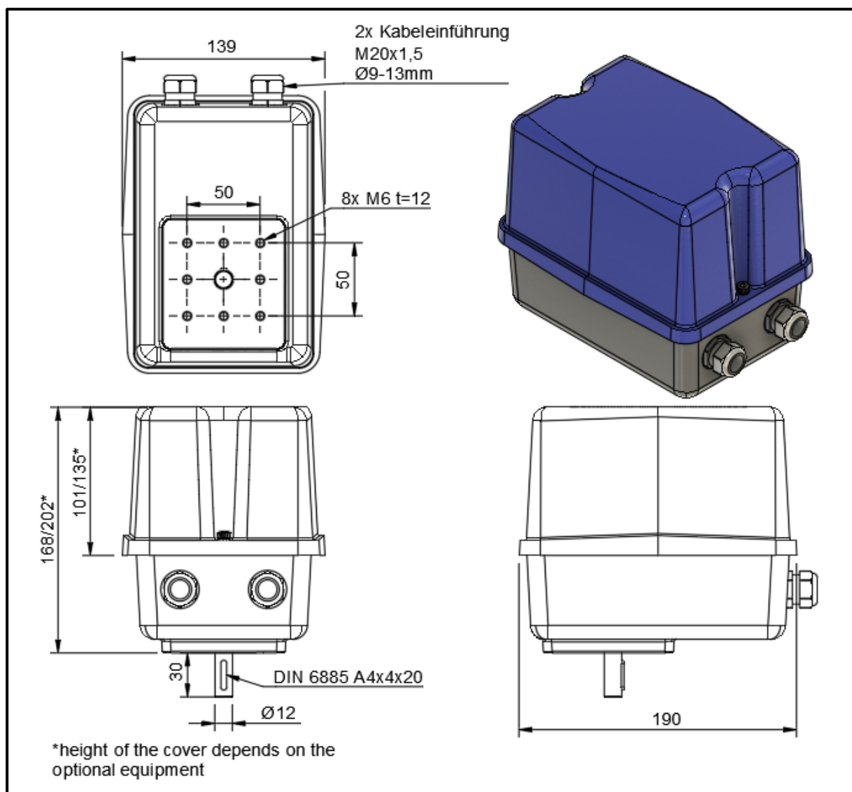
Abbildung 9: Abmessungen Antrieb Typ 02-25
