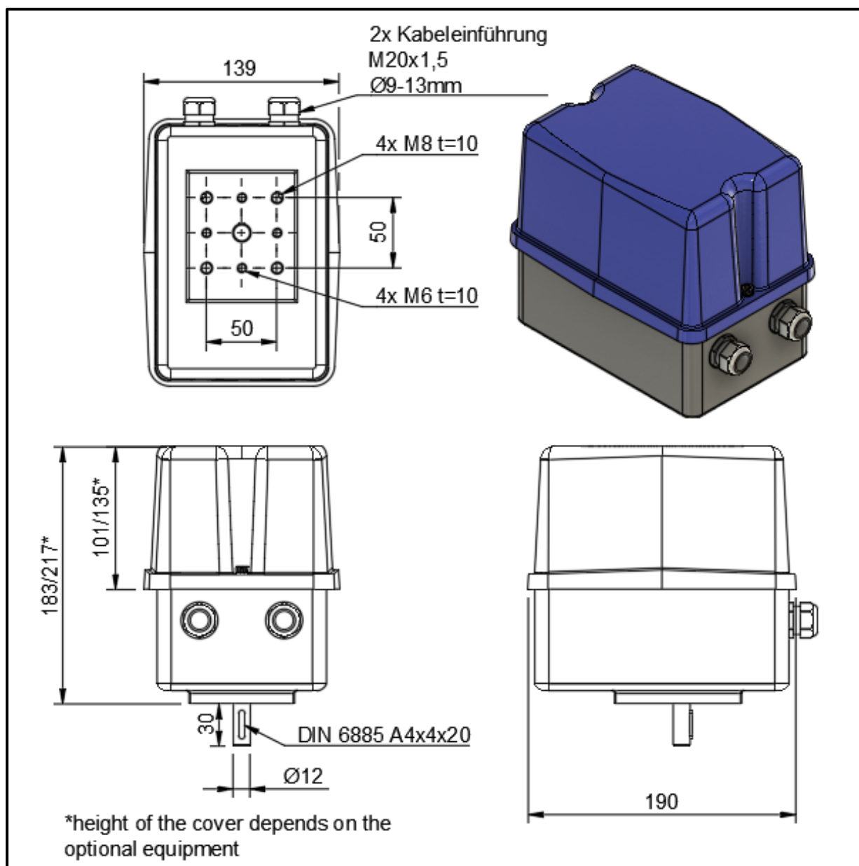
Abbildung 10: Abmessungen Antrieb Typ 02-50
