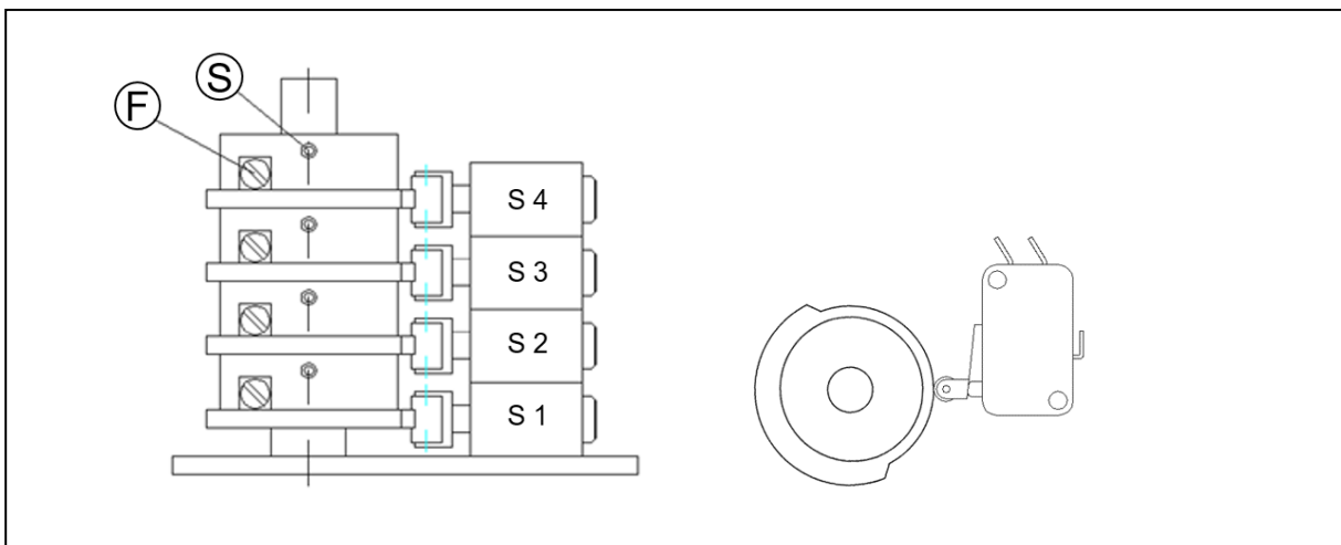
Abbildung 7: Nockenschalter inkl. 2 optionalen Zusatzschaltern
