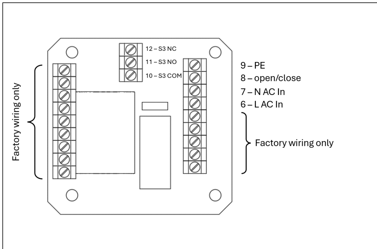
Abbildung 4: AB177 Anschlussbild, Version mit 1 Zusatzschalter
