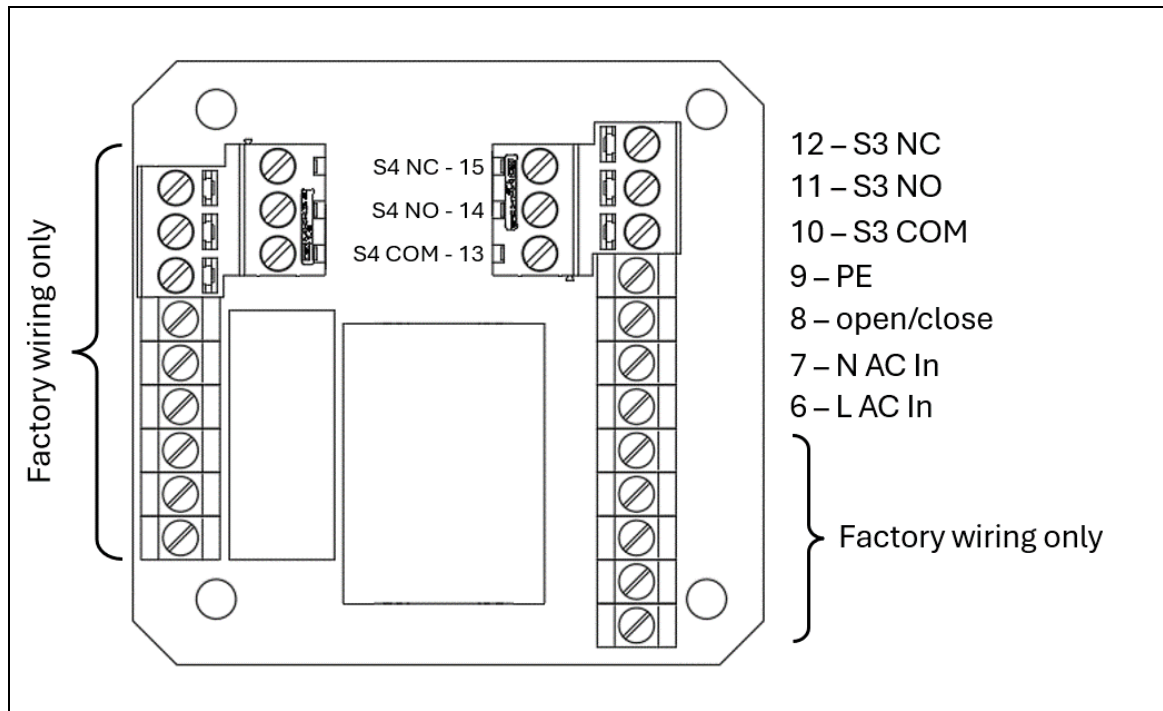
Abbildung 5: AB177 Anschlussbild, Version mit 2 Zusatzschalter
